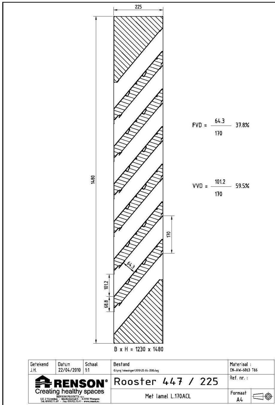
Bild 1 Senkrechter Querschnitt
